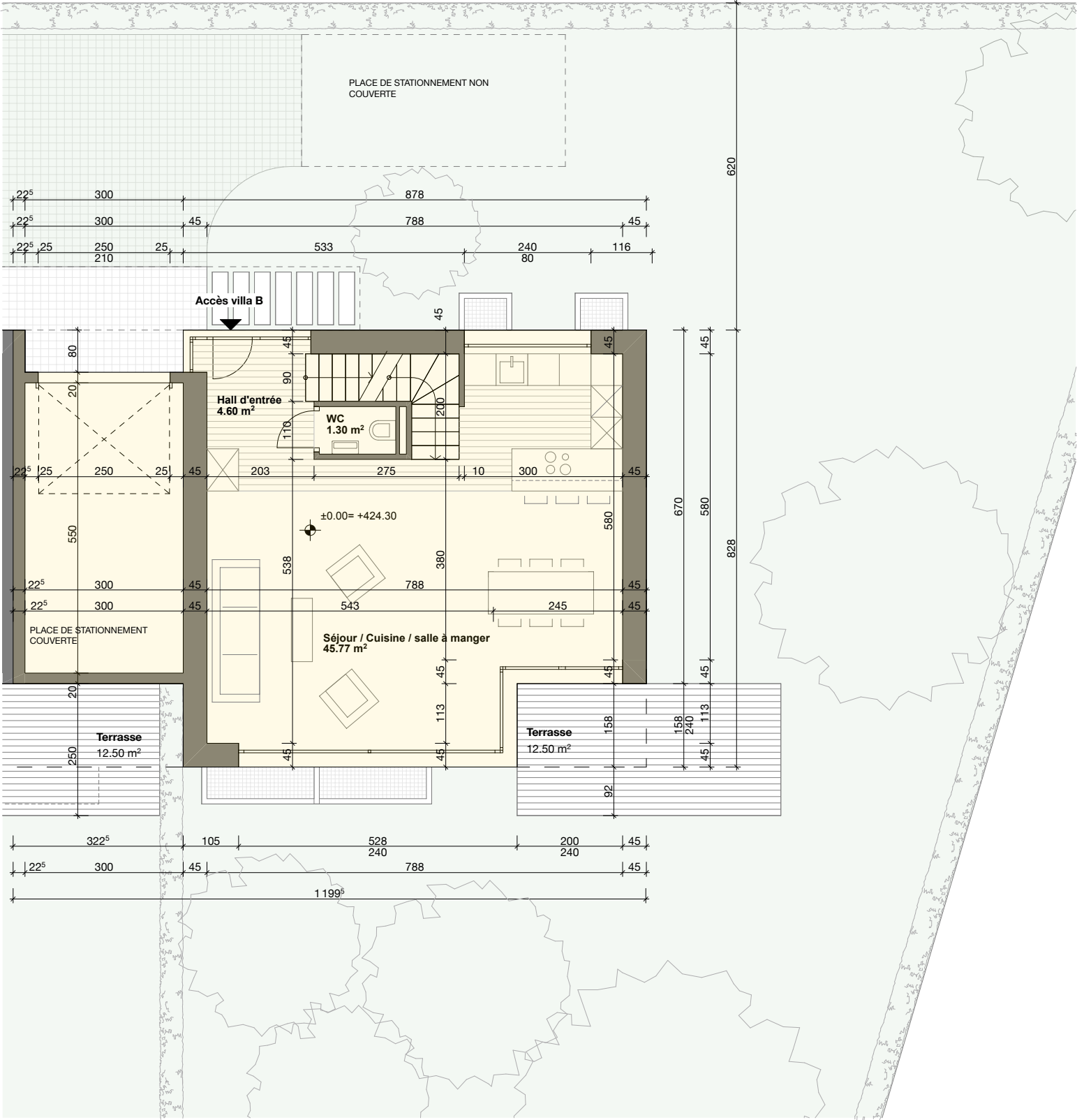
REZ-DE-CHAUSSÉE VILLA B
