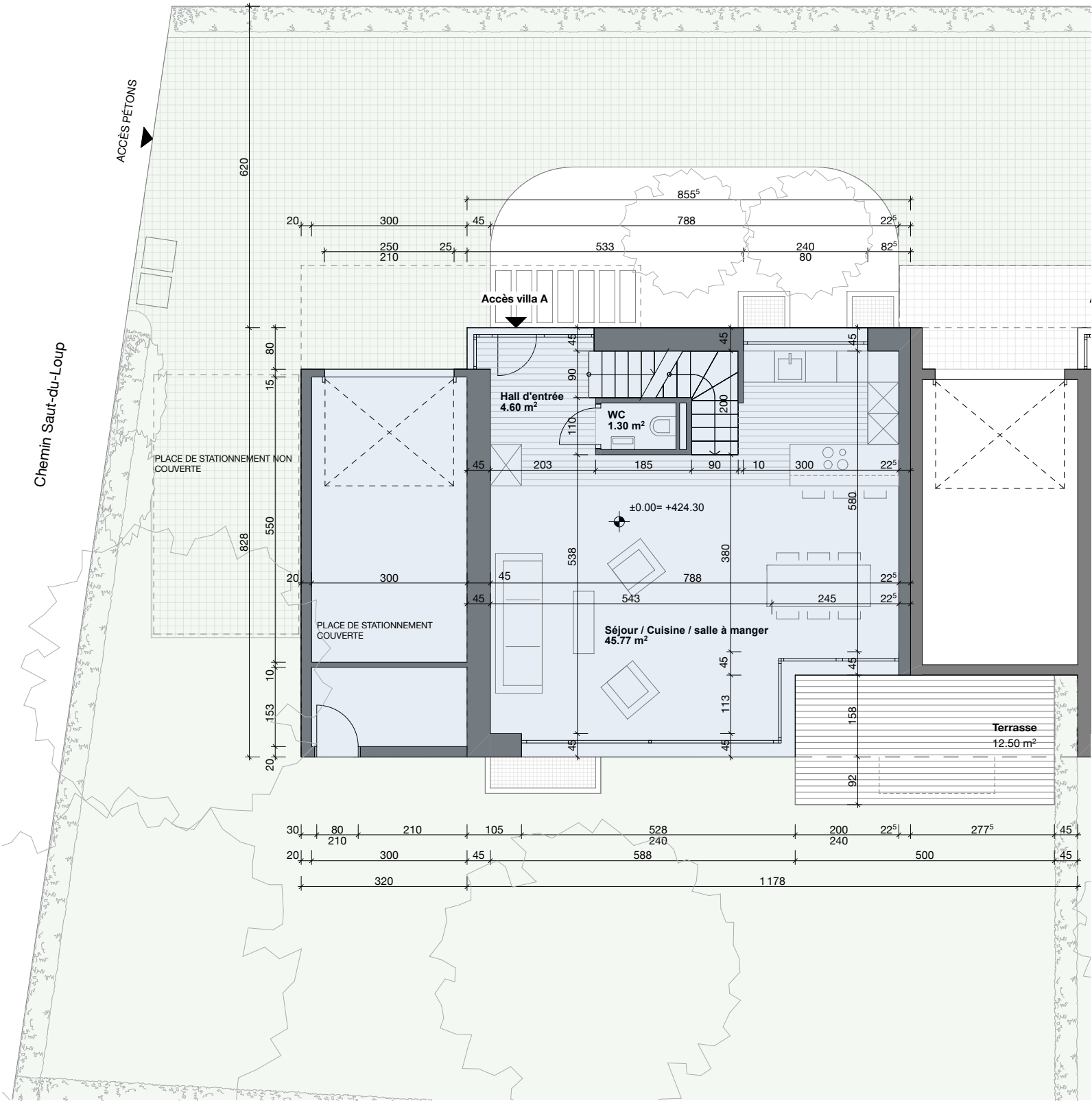
REZ-DE-CHAUSSÉE VILLA A
