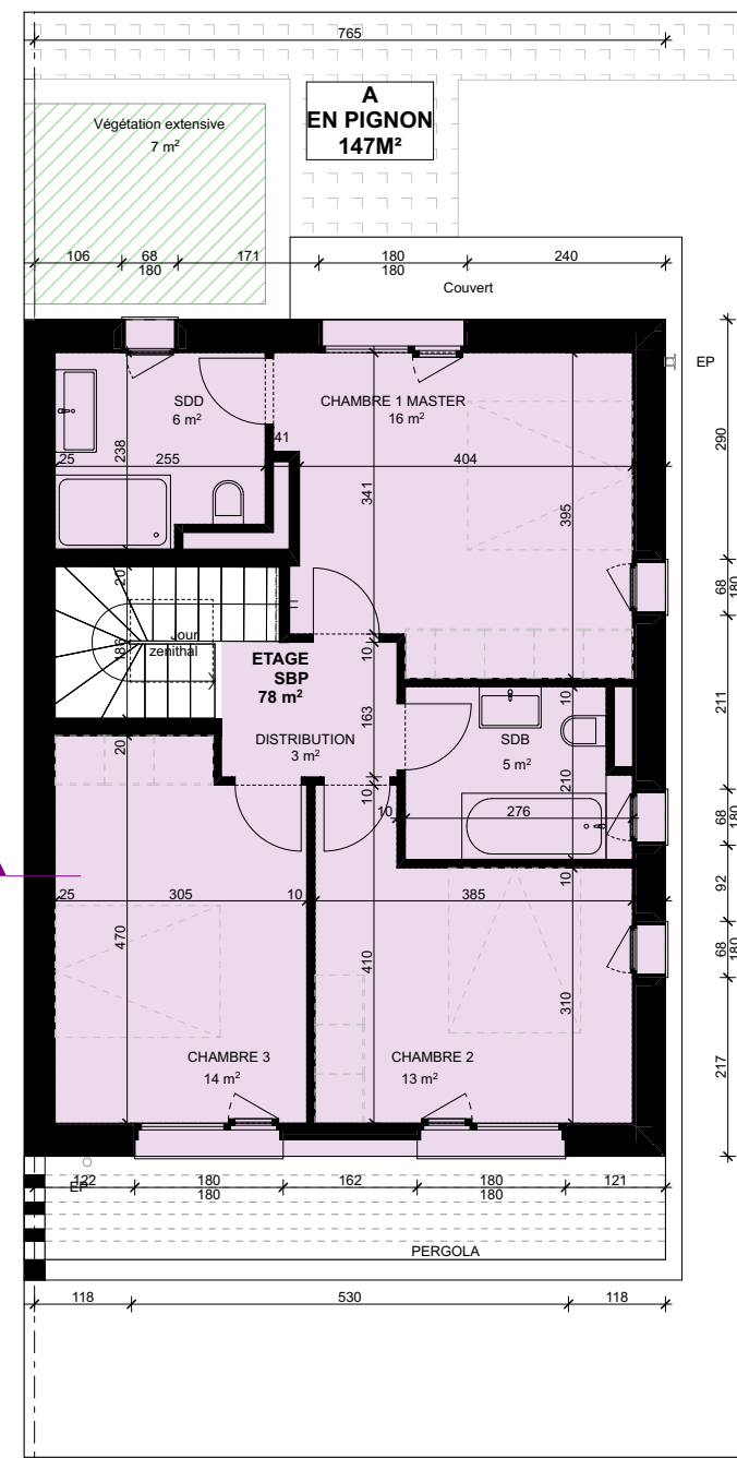
PLAN ETAGE
