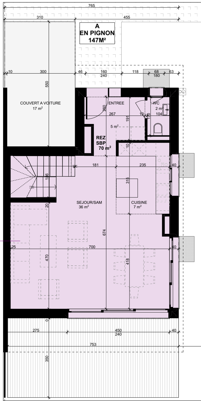
PLAN REZ DE CHAUSSEE
