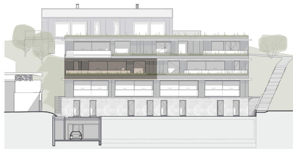
Elévation Sud
